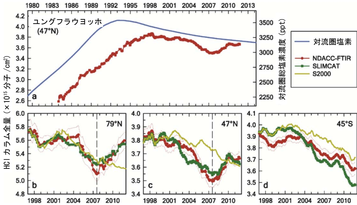
図 2. 大気中の HCl カラム全量の経年変化。図 a はユングフラウヨッホ(スイス)で観測された HClカラム全量の経年変化(赤線、3 年間の移動平均をかけた値を 1 ヶ月毎に表示、縦軸の数値は左側)と、全球平均の対流圏総塩素濃度(青線、縦軸の数値は右側)。下側の図は同じく移動平均をかけた HCl カラム全量の経年変化(1997-2011 年)で、図 b がニーオルスン(ノルウェイ)、図 c がユングフラウヨッホ、図 d がローダー(ニュージーランド)での値。それぞれ赤線は NDACC-FTIR 観測、緑線は SLIMCAT 標準計算、黄緑線は SLIMCAT の S2000 計算の結果。細い赤線は観測値に対する標準偏差の 2 倍で定義した誤差範囲。カラム全量の最低値は、北半球では波線で示す 2007 年 7 月に観測されている。[Mahieu et al./Nature]
