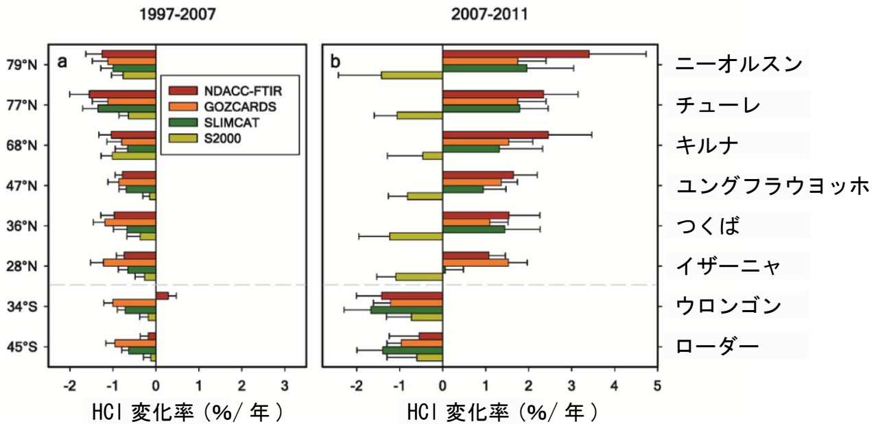
図 3. 8 つの NDACC 観測地点における HCI の変化率。図 a は 1997-2007 年の期間 (チューレ (グリーンランド) と イザーニャ (スペイン) については 1999-2007 年、つくばについては 1998-2007 年) における年変化率 (%/年)。図 b は 2007-2011 年の期間における年変化率。年変化率は FTIR および GOZCARDS (人工衛星) 観測データ、ふたつの SLIMCAT 計算結果から導出。エラーバーは標準偏差の 2 倍で定義した誤差範囲を示す。[Mahieu et al./Nature]
