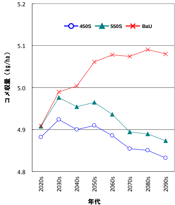
図Ⅱ-5-1 コメ収量（全国平均）．2100 年まで毎年の割合を算定し 20 年間の平均値を表示
