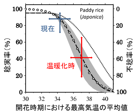
図Ⅱ-5-4 開花時期の気温と不稔率の関係
