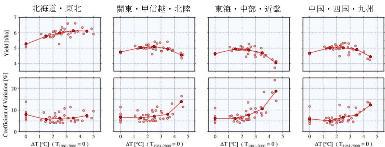
図Ⅱ-5-3 1981年～2000年の平均値に対する暖候期（5～10月）平均気温の上昇度に対する地域平均収量（上図）と変動係数の変化（下図）
