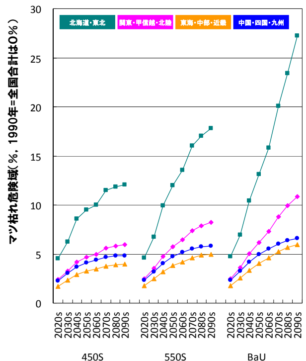
図 II-4-2 1990 年を基準とし、マツ枯れ危険域でない地域が危険域に変わっていく割合（地域別）。2100 年まで毎年の割合を算定し 20 年間の平均値を表示
