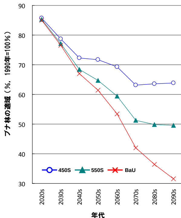
図Ⅱ-3-1 1990 年を基準(100%)とした場合のブナ林の適域変化（全国平均）。2100 年まで毎年のブナ林の適域を算定し 20 年間の平均値を表示
