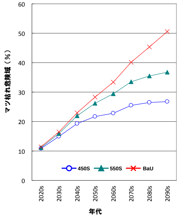
図 II-4-1 1990 年を基準とし、マツ枯れ危険域でない地域が危険域に変わっていく割合（全国平均）。2100 年まで毎年の割合を算定し 20 年間の平均値を表示
