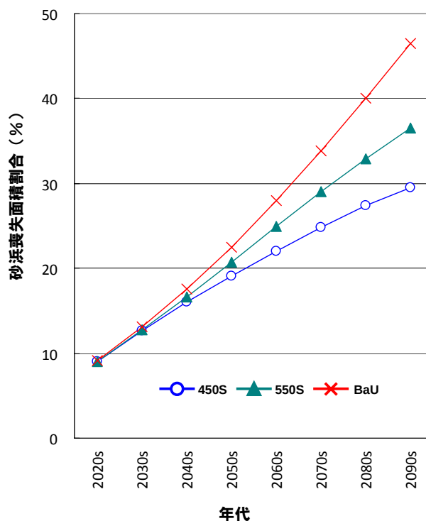
図Ⅱ-6-1 砂浜喪失割合(全国平均)。2100 年まで毎年割合を算定し 20 年間の平均値を表示
