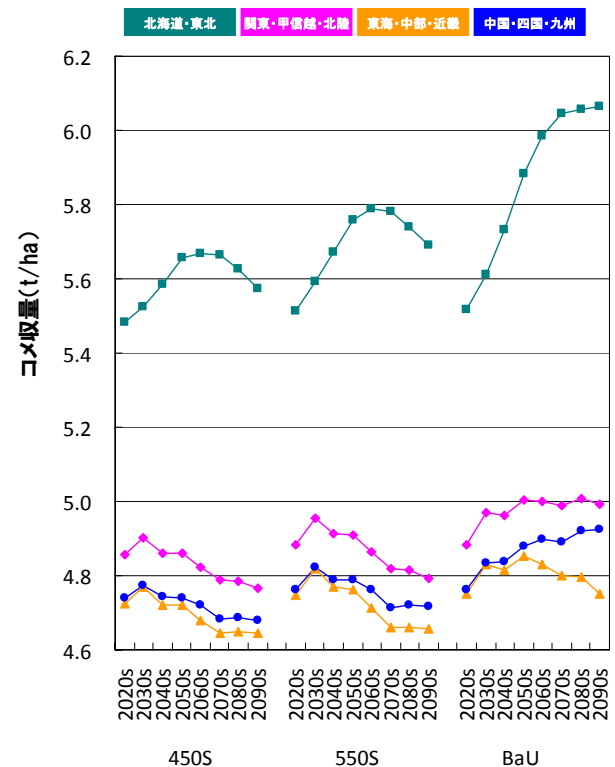
図Ⅱ-5-2 コメ収量（地域別）．2100 年まで毎年の割合を算定し 20 年間の平均値を表示
