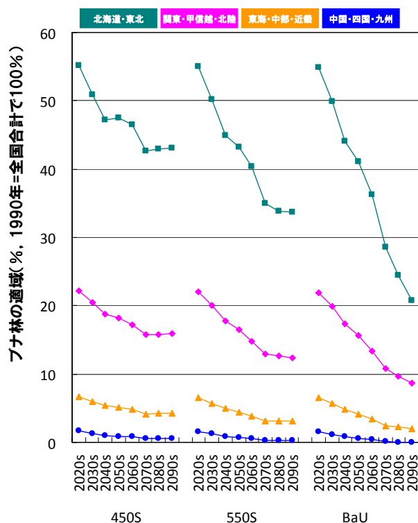
図Ⅱ-3-2 1990 年を基準(100%)とした場合のブナ林の適域変化（地域別）。2100 年まで毎年のブナ林の適域を算定し 20 年間の平均値を表示
