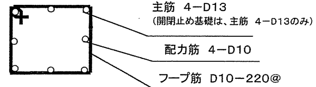
支柱部鉄筋平面図
