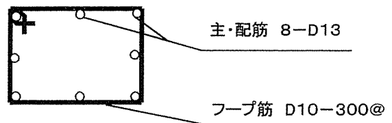
基礎部鉄筋断面図
