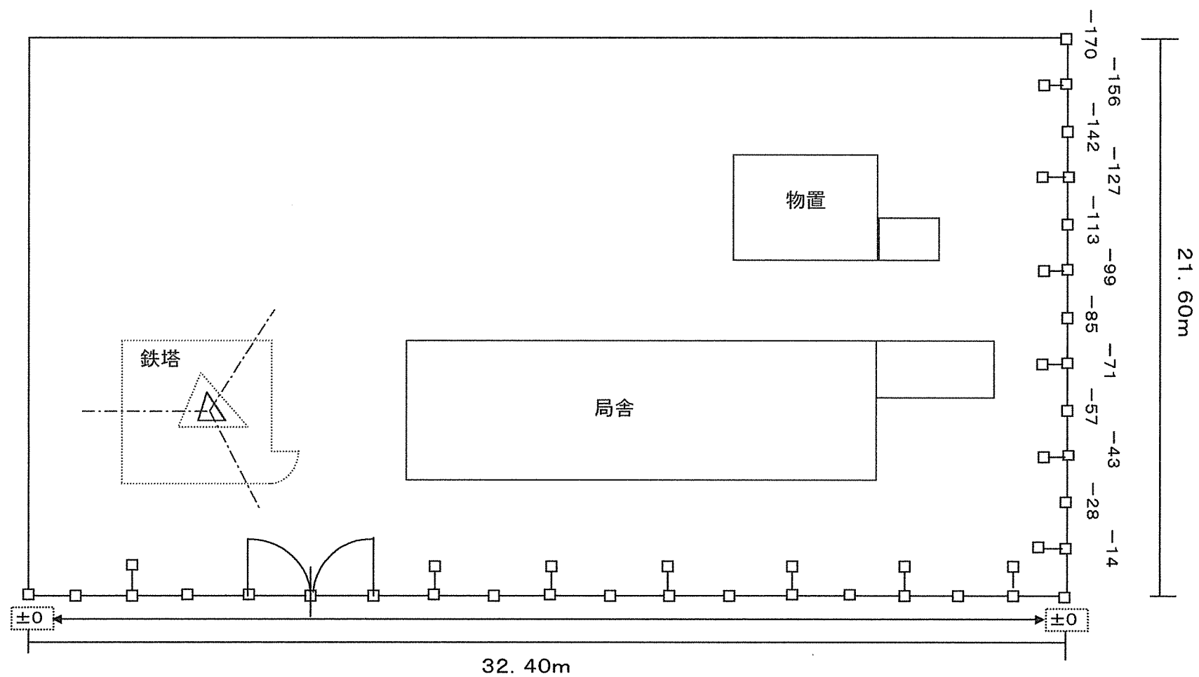
フェンス基礎レベル図
