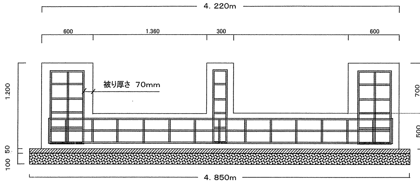
基礎部鉄筋平面図
