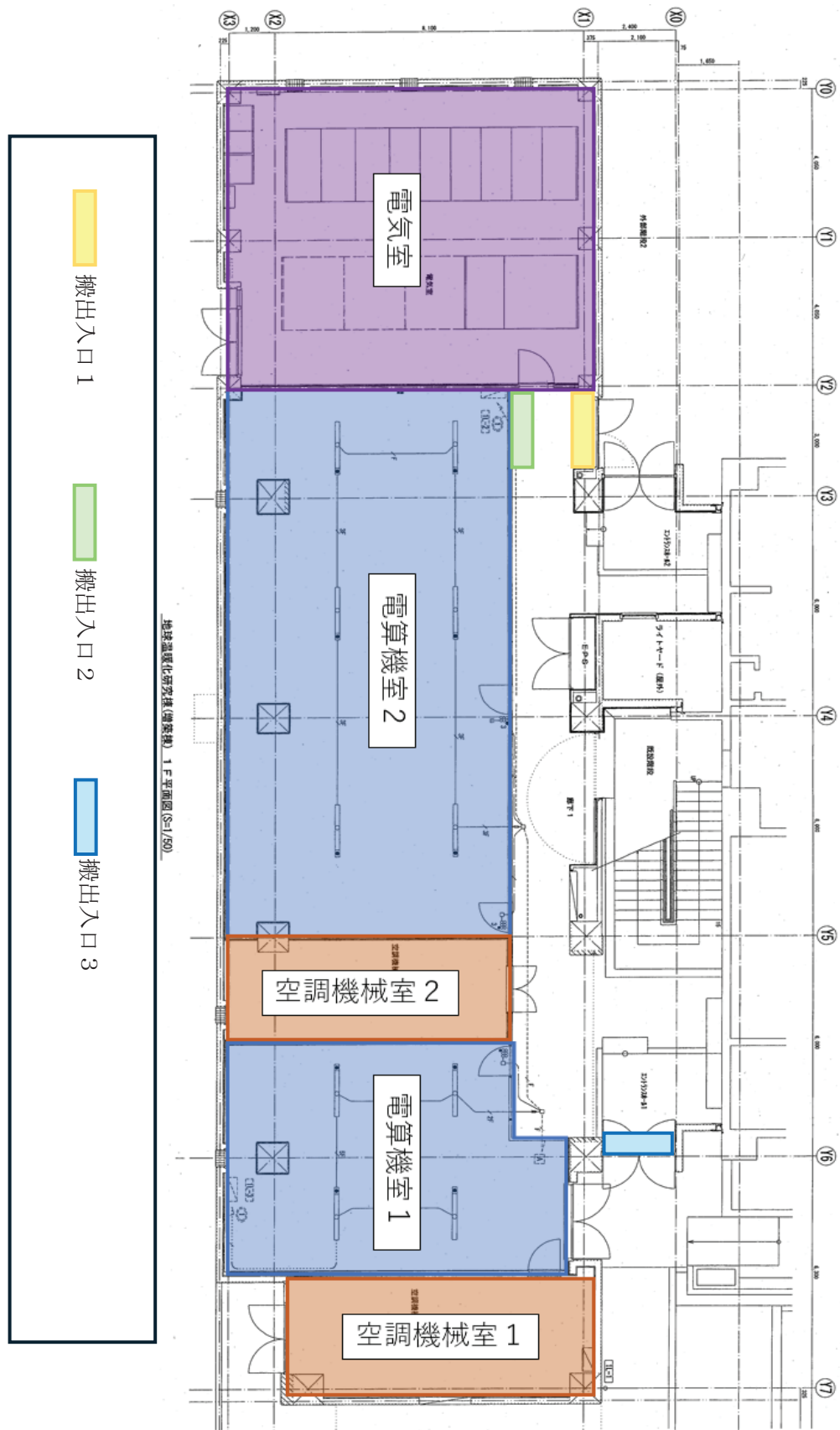
(図1) 地球温暖化研究棟増築部の見取り図
