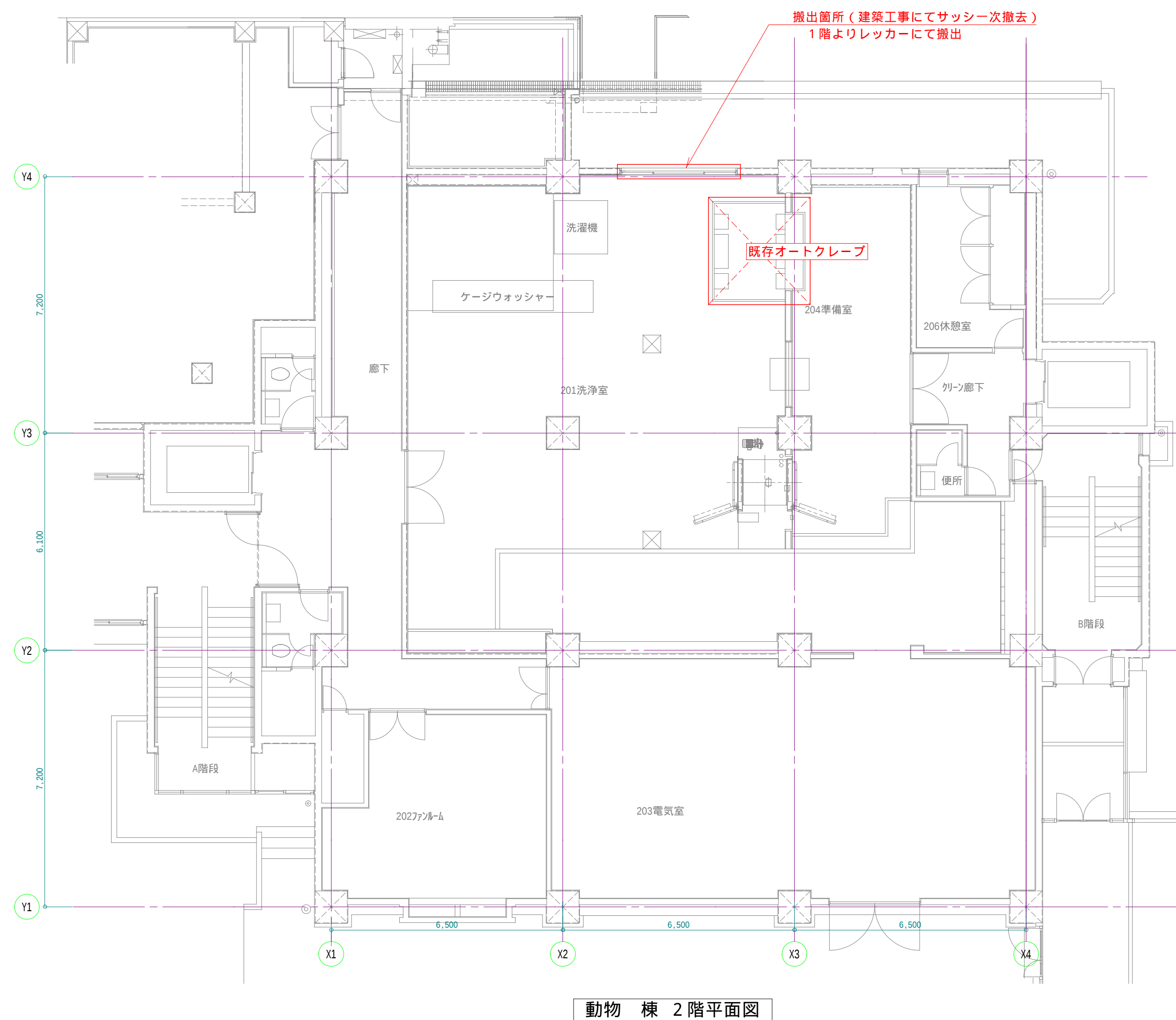
動物棟 2階平面図
