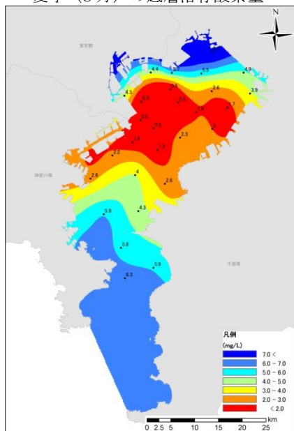
平成 19 年度 夏季（8 月）の底層溶存酸素量
