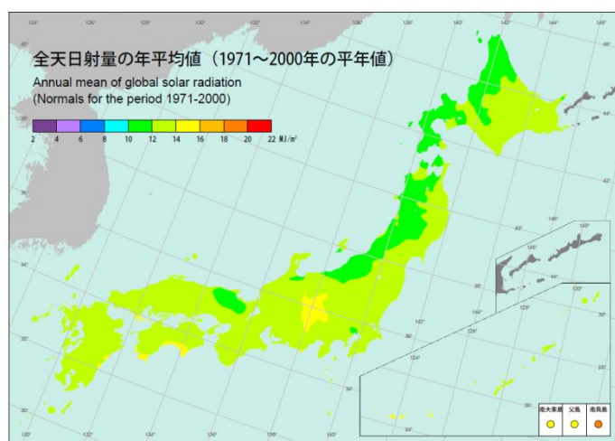
図 24 我が国の全天日射量年平均值の分布 (1971 年～2000 年平均値)
