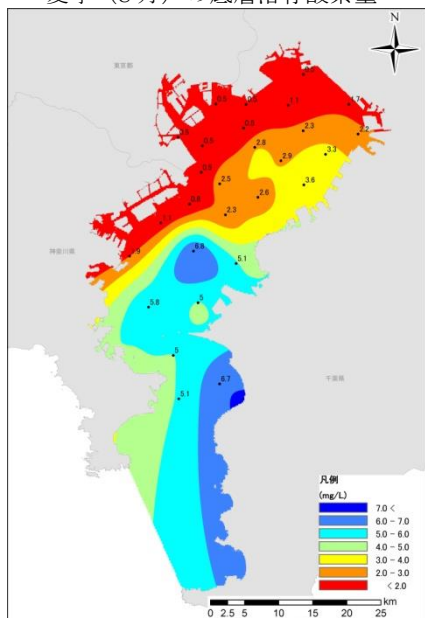
平成 18 年度 夏季（8 月）の底層溶存酸素量
