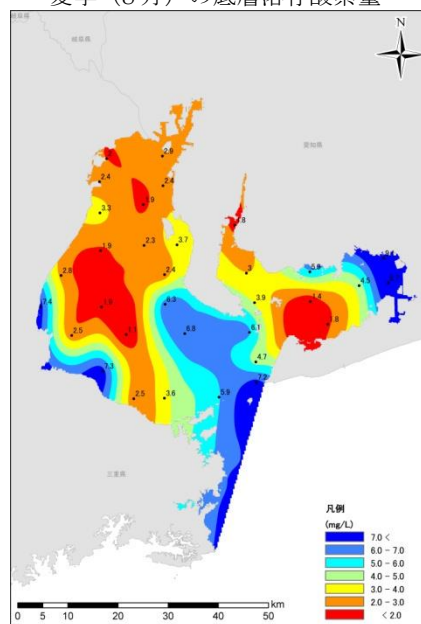
平成 20 年度 夏季（8 月）の底層溶存酸素量
