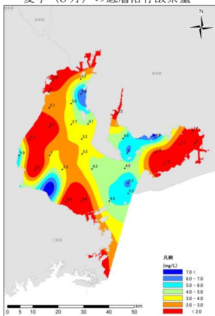
平成 18 年度 夏季（8 月）の底層溶存酸素量
