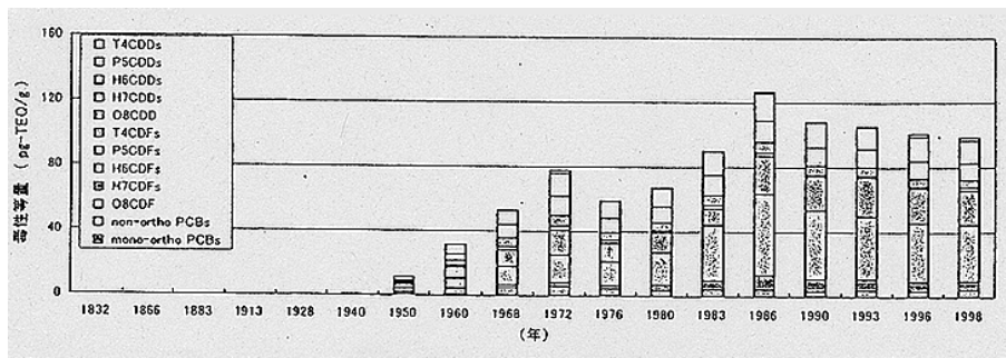
各地点のPCDD+PCDF+Co-PCB測定結果(毒性等量)
