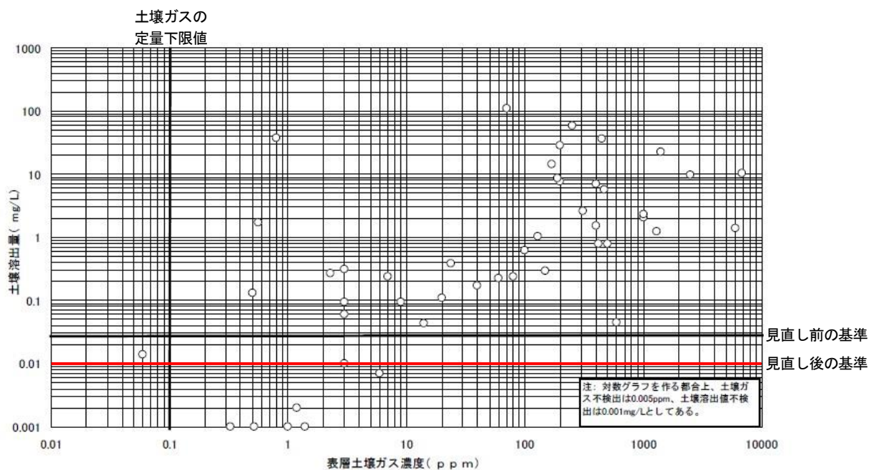
図1 表層土壌ガス濃度と土壌溶出量の関係（トリクロロエチレン） 土壌汚染対策法に係る技術的事項について（答申）（平成14年中央環境審議会）
