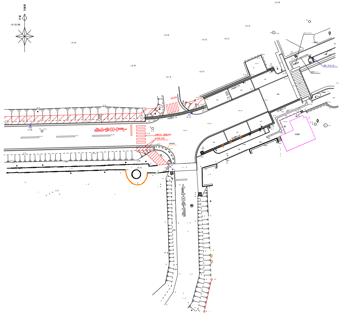
守衛所付近 更新図
