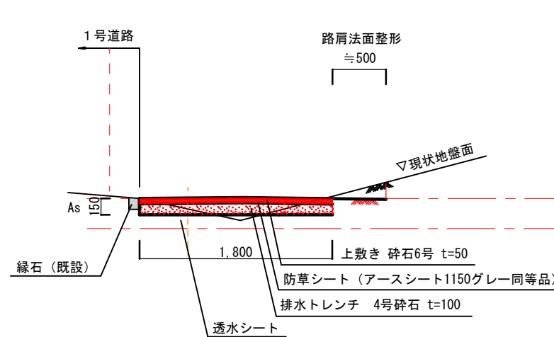
C-C' 横断面図
