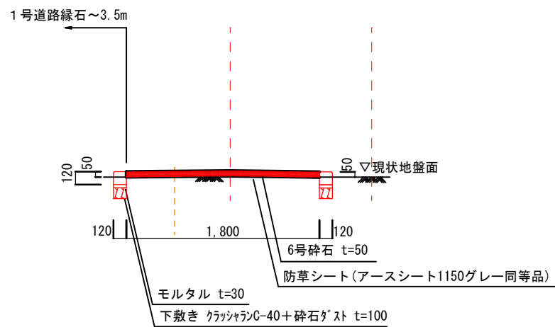
A-A' 断面図
