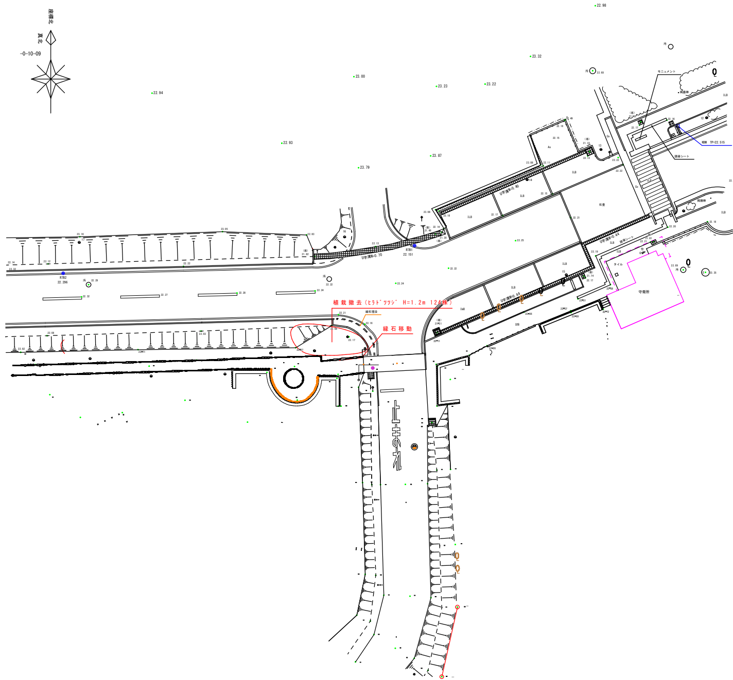
守衛所付近 撤去図
