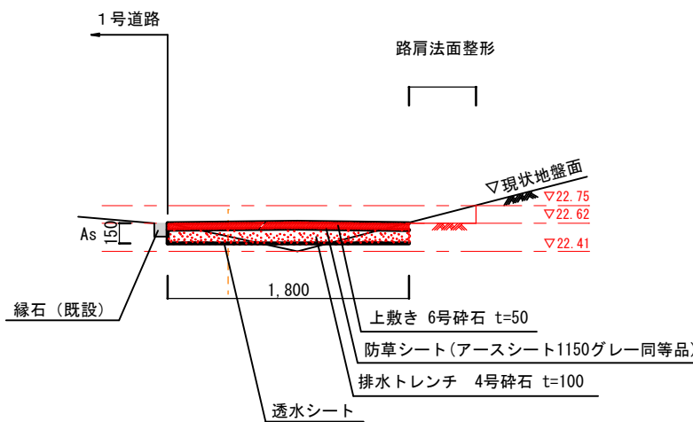
B-B' 断面図
