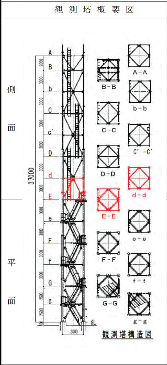
観測塔の劣化箇所② 欠損箇所の貫通あり
