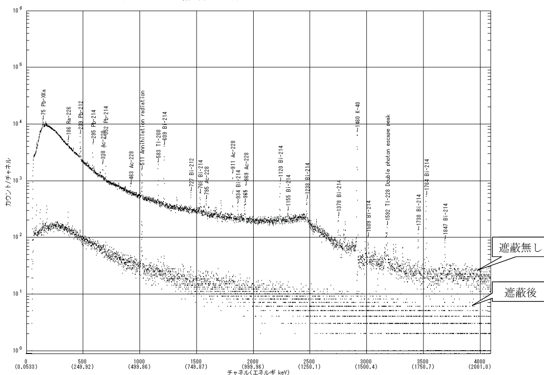
図6. 遮蔽前後の Ge \gamma 線検出器のバックグラウンド（測定時間 10 5 秒）
