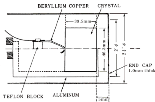
図 7. Ge \gamma 線検出器
