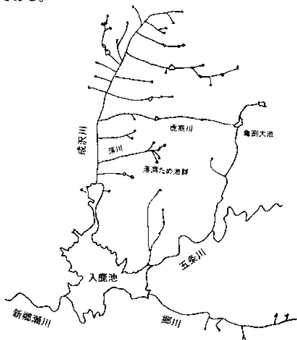
図 1 . 入鹿池とサテライトため池群.
