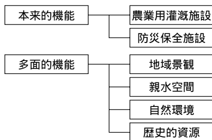
図1．ため池が有する機能。
