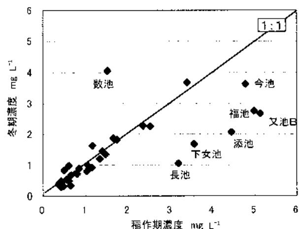
図6．ため池の稲作期 TN 濃度と冬期 TN 濃度の関係．
