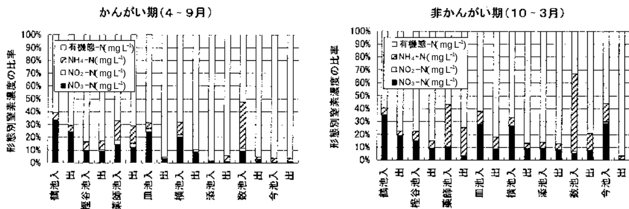
図3．ため池の形態別窒素濃度比率（％）.
