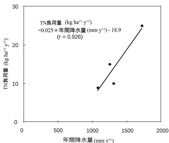
図 5 . 神戸における年間降水量とTN負荷量の関係.
