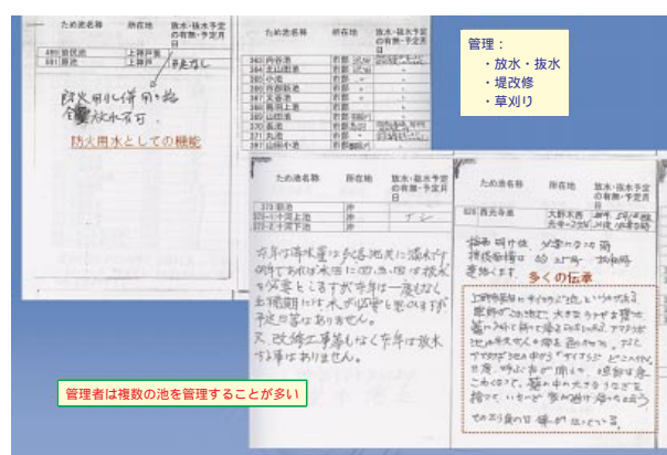
図 3．ため池の管理状況を管理者に往復ハガキで照会した結果の一例。
