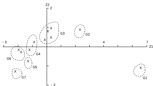
図3．因子得点.
