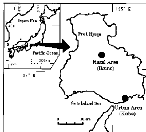
図 1 . 調査地点の概略図.
