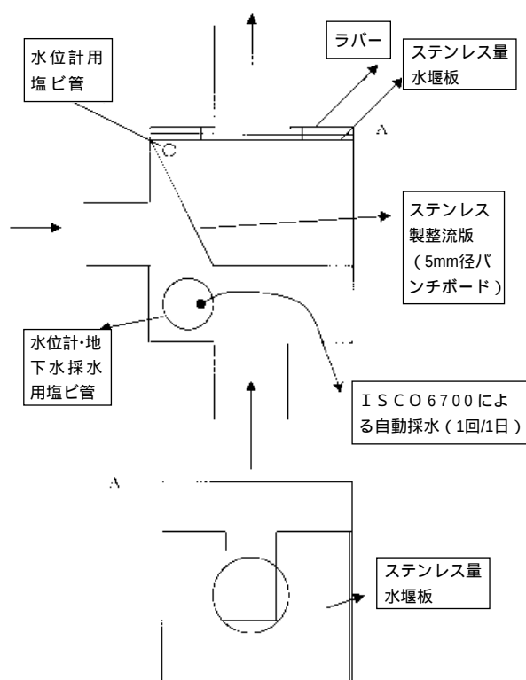
図．会所マス( # 32 ).
