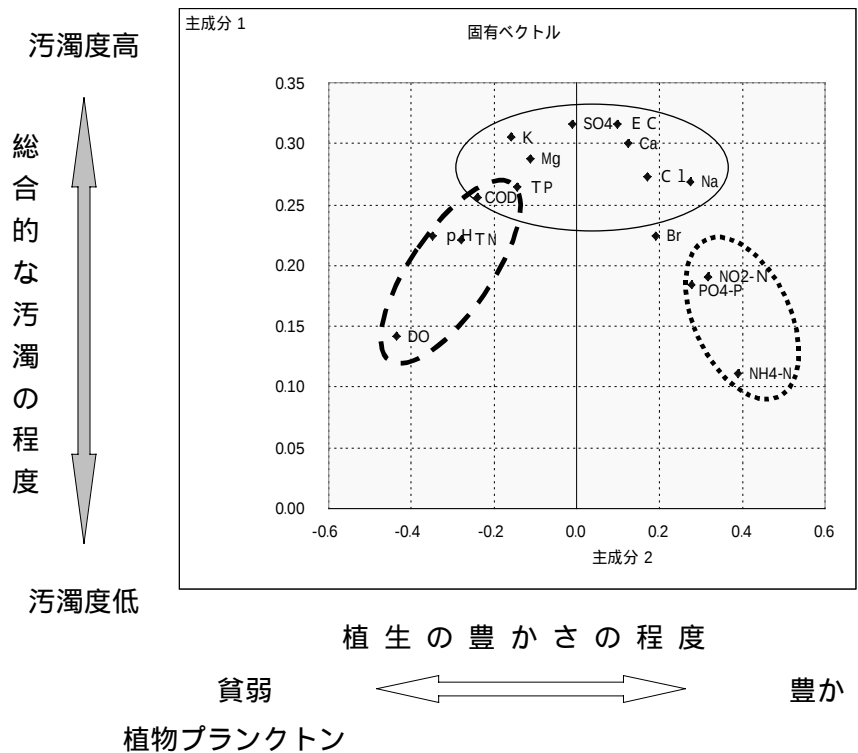
図 5 . かんがい期における水質分析項目の主成分分析結果.
