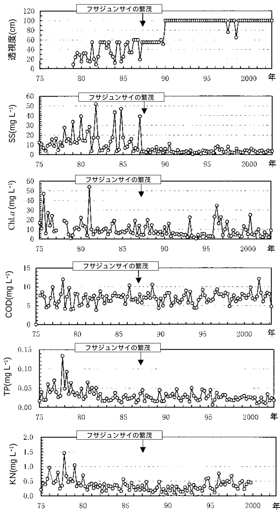
図3 . 塚の杓池における水質の変遷(1975～2002年)
