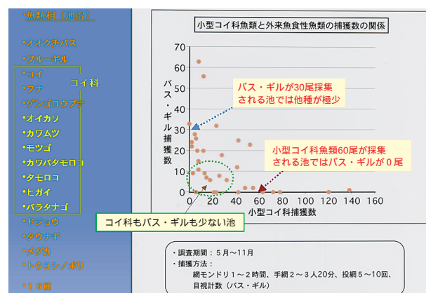
図 4．三重県上野市における溜め池の魚類相。
