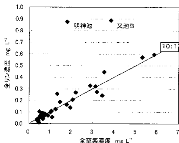
図5．ため池の全期平均 TN 濃度と TP 濃度の関係．
