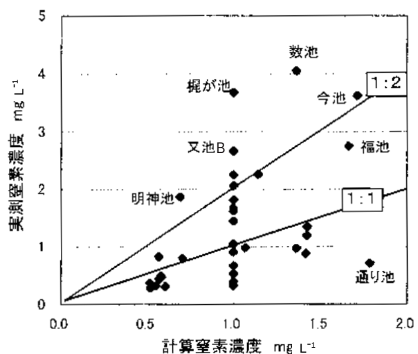
図8. ため池の計算濃度 X_{cn} と実測濃度 X_{pn} の比較(非稲作期 TN)
