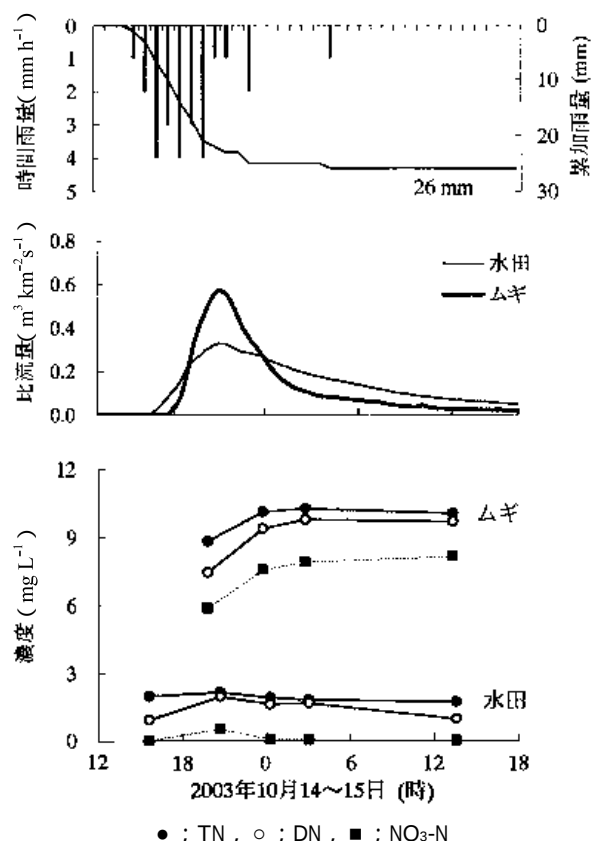
図7. 降雨(26mm)時の排水量と窒素濃度 に与えるムギ転作の影響。
