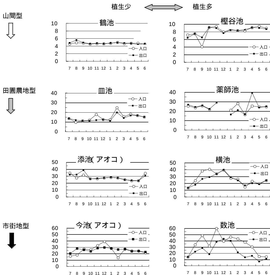
図2．ため池におけるECの季節変動 単位( mS m -1 ). ○ : 入口 ■ : 出口
