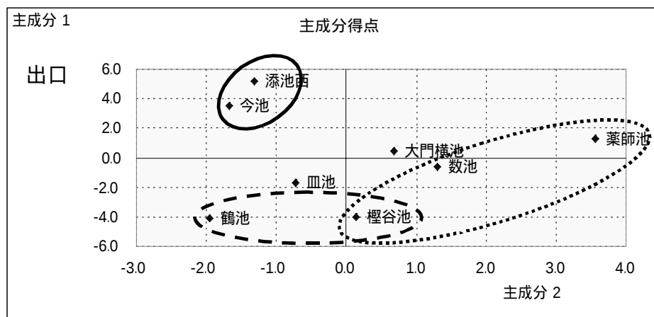
図 6 . かんがい期におけるため池の主成分得点分布 .
