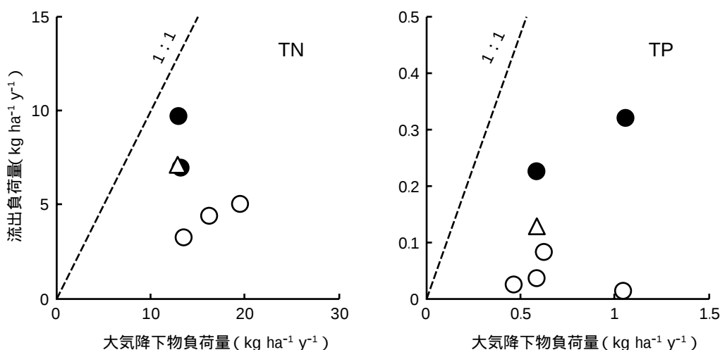
図3．森林の大気降水物負荷量と流出負荷量との関係．
