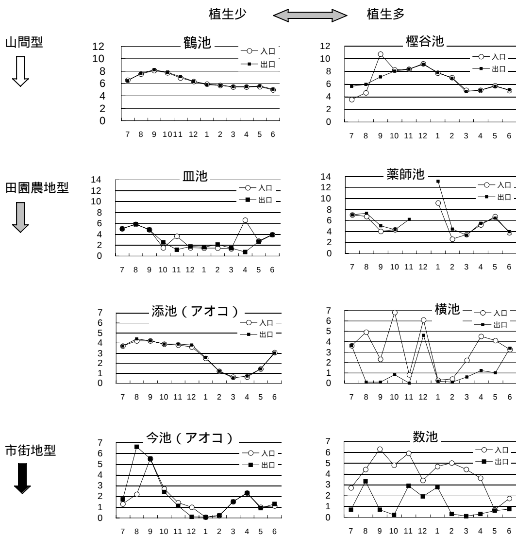
図4．ため池におけるケイ素濃度の季節変動 単位( \text{mg L}^{-1} ). ○：入口 ■：出口
