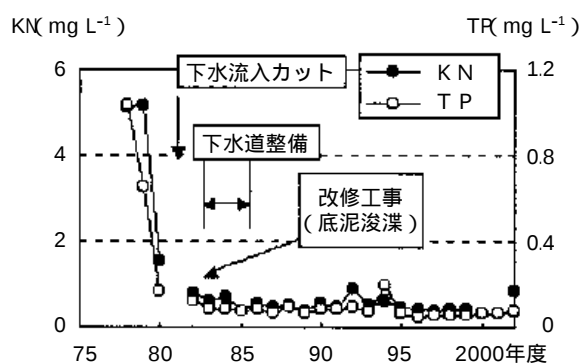
図 3-8 . 螺貝池の経年変化.
