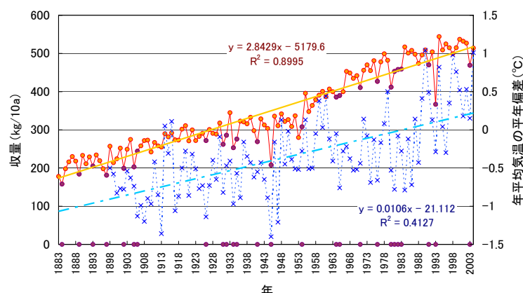
図 I-III-7 水稻収量および年平均気温の変動
