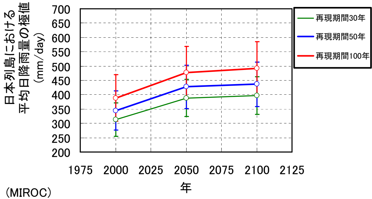
図 I-I-2 MIROC による近未来(2030-2050 年)と 2100 年頃(2080-2100 年)の降雨の状態。20 年間の日本全域の値の平均値と分散値(縦線)を示す
