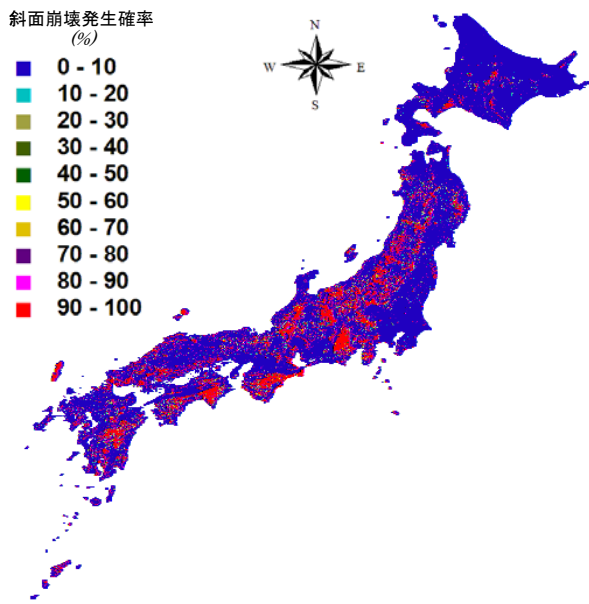
図 I-I-5 2050 年気候時の 30 年に 1 回生じるとされる豪雨による斜面崩壊発生確率。豪雨の発生確率は不確実性が高く、この結果はやや過大な結果といえる
