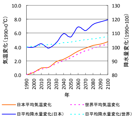
図 1 日本域および全球における 1990 年～2100 年の気温上昇および降水量変化 (MIROC)
