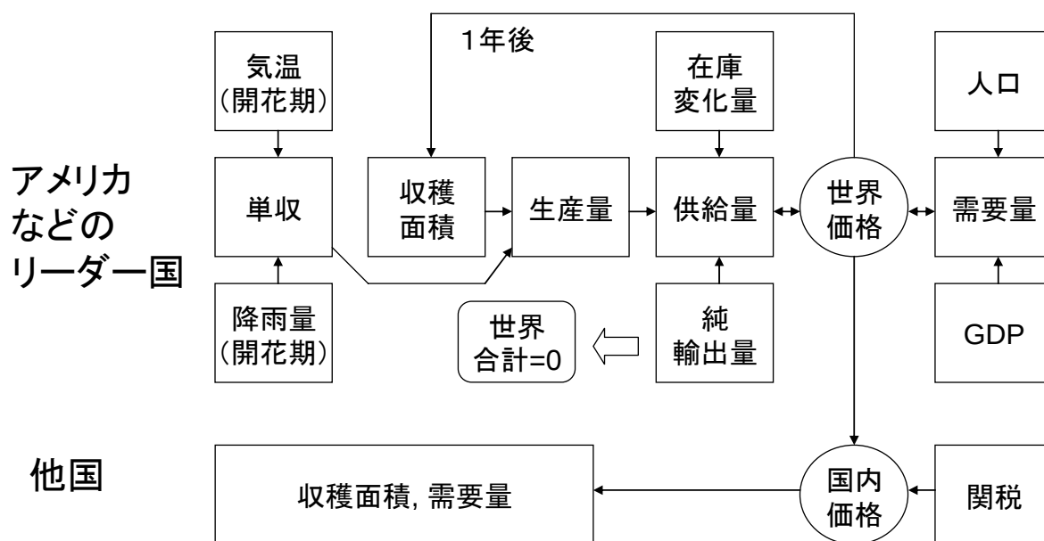
図 I-III-3 世界食料モデルの作物部門の構造
