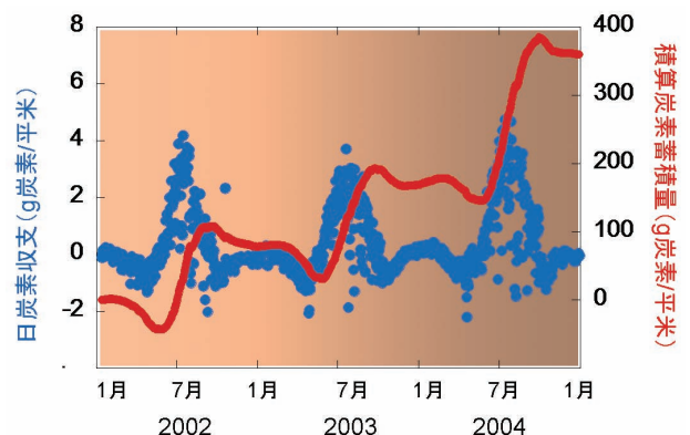
図 青海草原の炭素収支
