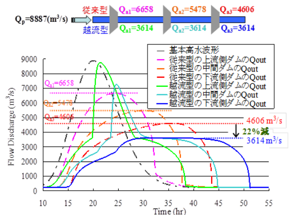
図 2(2)-8 カスケード方式による洪水制御能力
