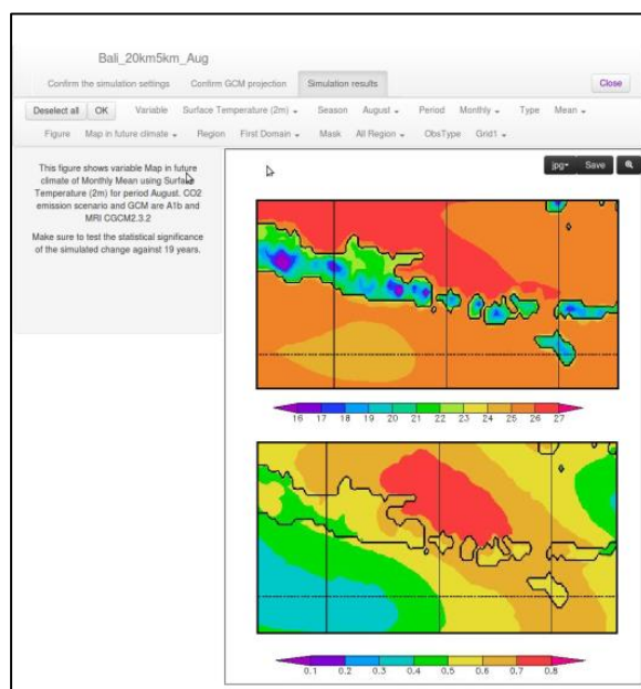
図 1(2)-4 ダウンスケーラから得られた将来予測の月平均の地上気温分布 (上) と将来と現在の月平均の地上気温の差の分布 (下) の図。対象領域はインドネシア、解像度は 20km、計算期間は 1981-2000 年および 2031-2050 年の 8 月、GCM は MRI CGCM 2.3.2、排出シナリオは SRES A1b。
