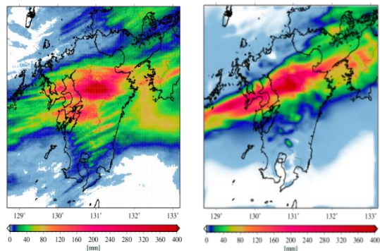
図 2(2)-5b 平成 24 年 7 月九州北部豪雨の 12 時間積算雨量分布 (左: レーダーアメダス解析雨量, 右: シミュレーション結果)
