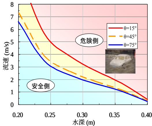
図 2(2)-9 冠水時の車走行危険判読図
