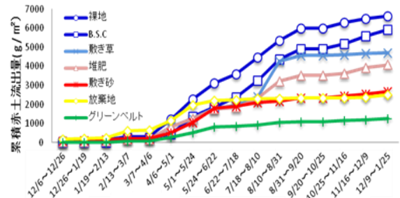
図 2(2)-7 適応策による赤土流出抑制効果
