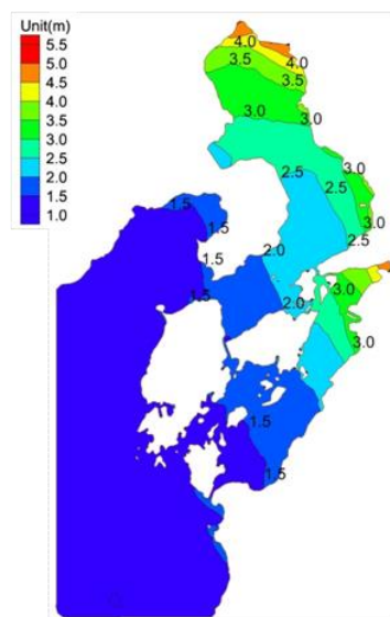
図 2(2)-6 将来気候による最大高潮偏差分布
