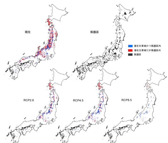
図1(5)-2. 現在気候と3つのRCPの将来気候シナリオで予測されたブナの潜在生育域と自然保護区の比較。現実的な評価を行うため、ブナの潜在生育域は、実際の分布域内に限定してある。
