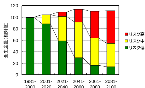
図 1(6)-1 全生産量の 20 年毎の推移 (MIROC3.2-hires A1b; 適応なし) 各メッシュの算定収量に水田面積を乗じて全国集計したもので、1981-2000 の現行移植日による値を 100 とした場合の相対値で表した。高温に因る品質低下のリスク：低(HDD<20)、中(20<HDD<40)、高(40<HDD)
