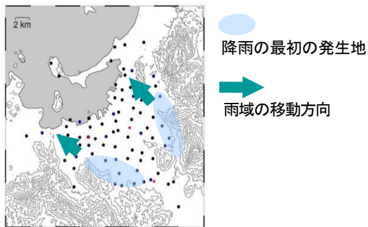
図 2(2)-5a 局地降雨の発生と雨域の移動の模式図
