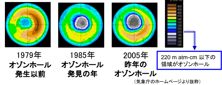
南半球のオゾン全量分布(10月の平均値)
